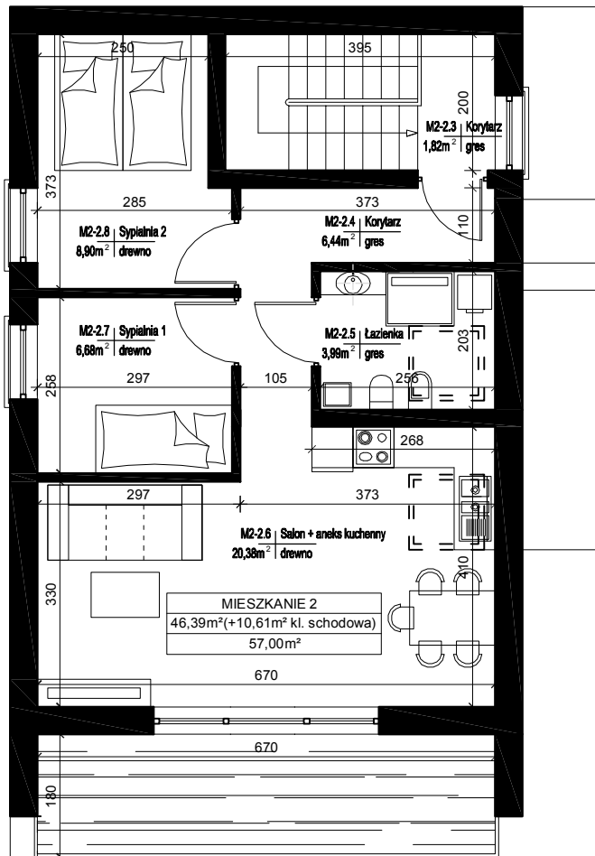
RZUT PODDASZA
